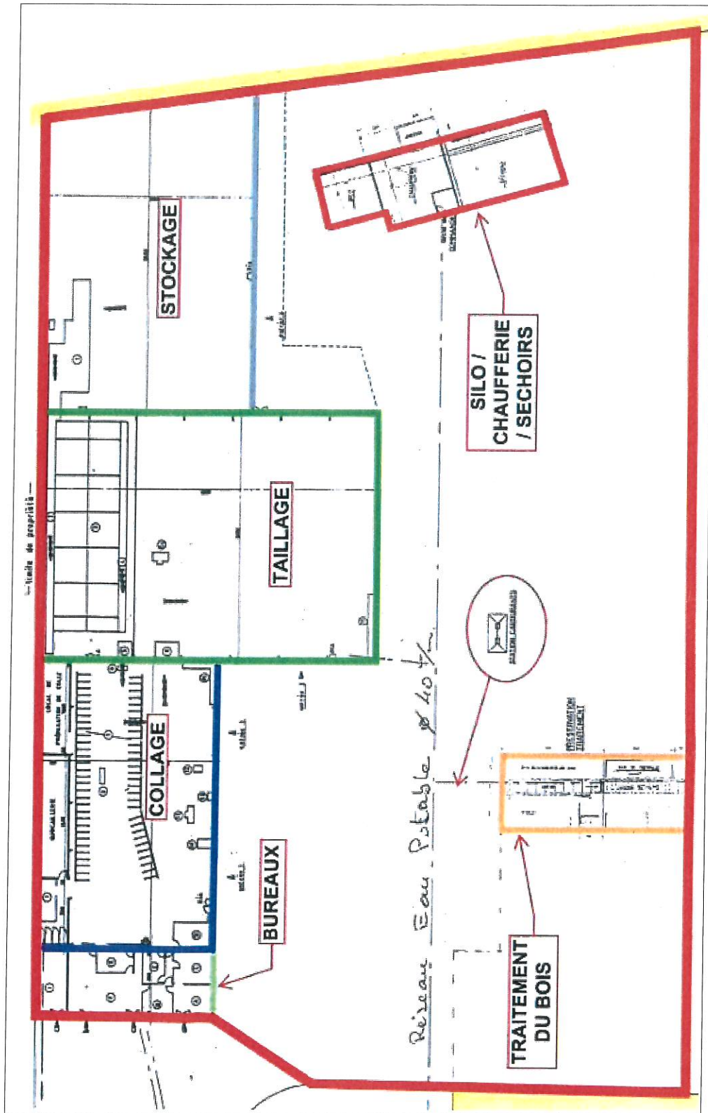
Plan de masse des installations Cormenier à Saint-Claud (16)
